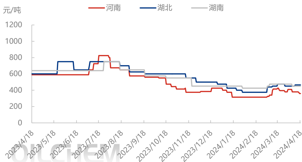
图表 6 华中地区分省份液氧价格走势
