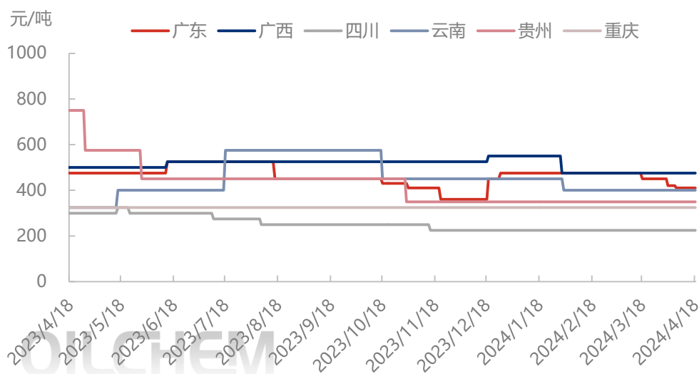
图表 8 华南西南地区分省份液氧价格走势图
