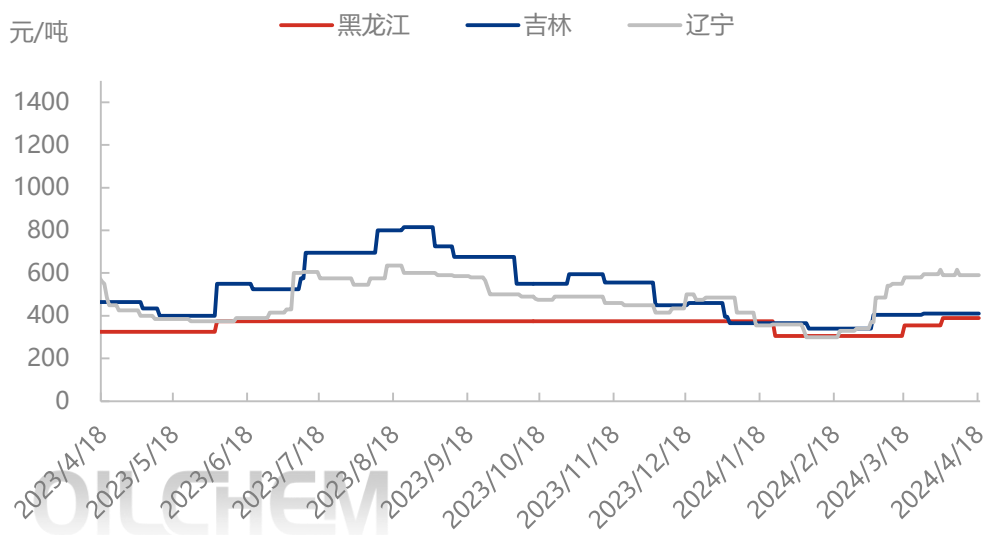
图表 4 东北地区分省份液氧价格走势
