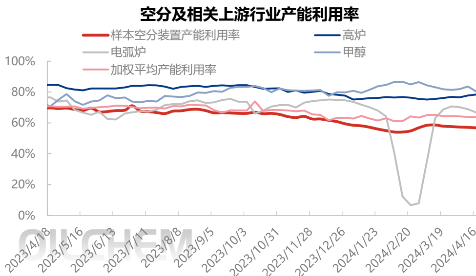
图表 11 国内样本空分产能利用率走势图
