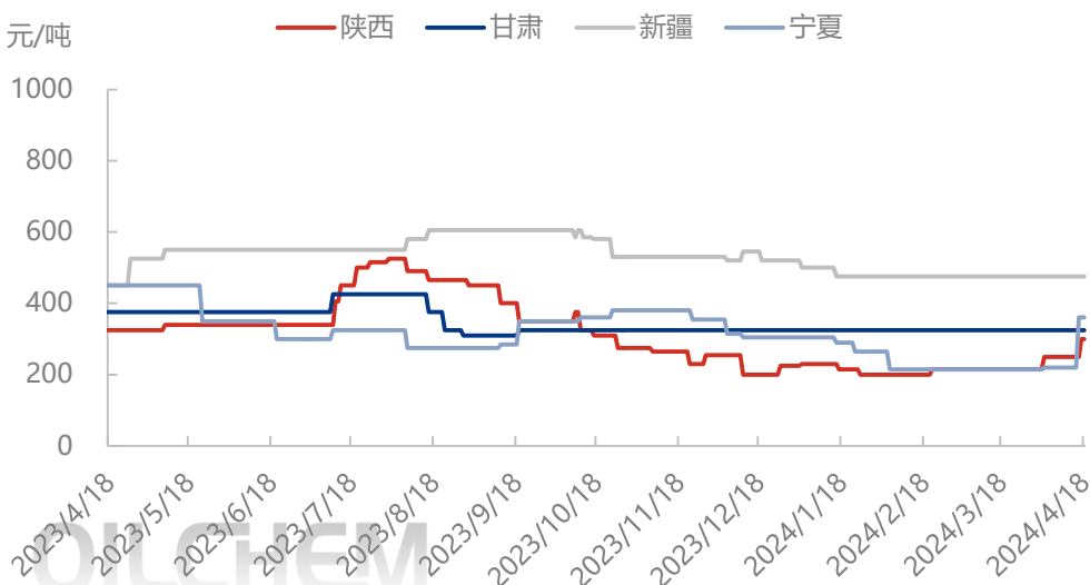
图表 9 西北地区分省份液氧价格走势图
