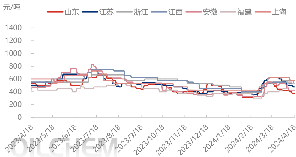
图表 7 华东地区分省份液氧价格走势
