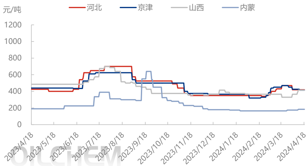
图表 5 华北地区分省份液氧价格走势
