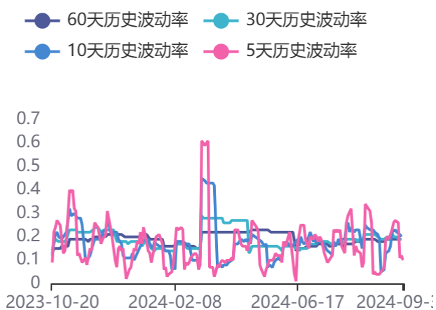
图67：历史波动率
