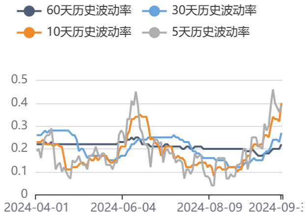
图77：历史波动率
