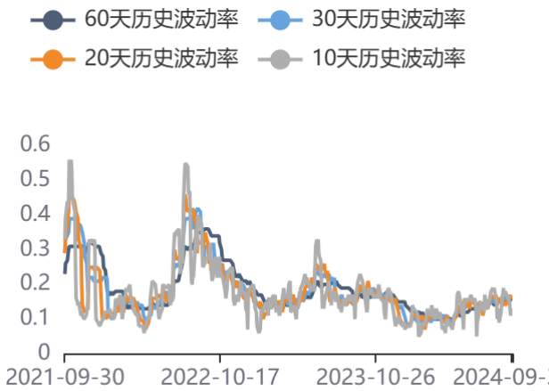
图82：历史波动率
